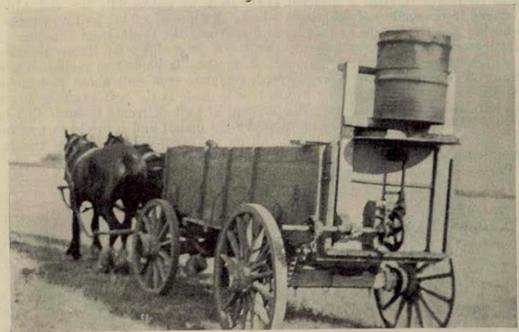
FIG. 3.—Endgate bait spreader.
